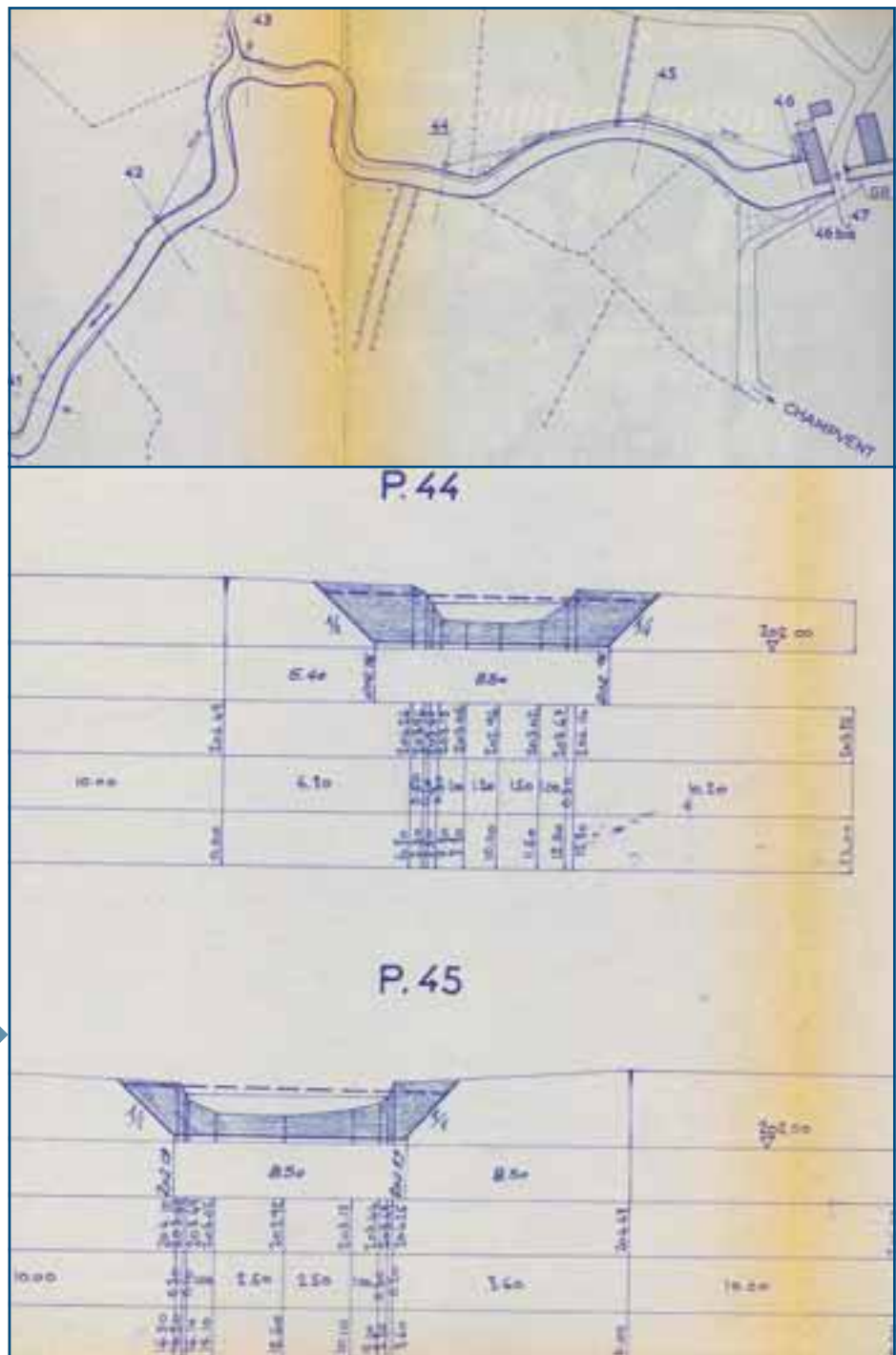
Figure 24 : Exemple de projet de recalibrage généralisé d'un cours d'eau. En blanc le profil initial, en gris le profil à créer (source DDAF 01). ≡
